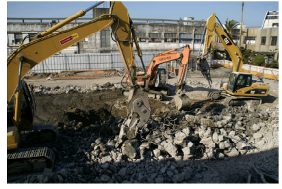
〈 第2棟跡地と、重機によるコンクリート破砕作業 〉
